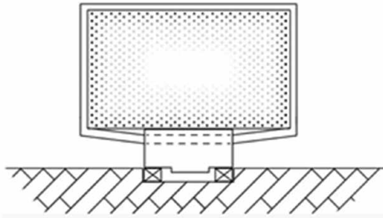
Obr. 2: Vertikálny rez saní a „koľajníc“ (nosníkov) použitých na prepravu kameňa
