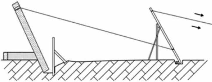
Obr. 1: Konštrukcia v tvare 'A' použitá ako páka na vztýčenie bloku do zvislej polohy
