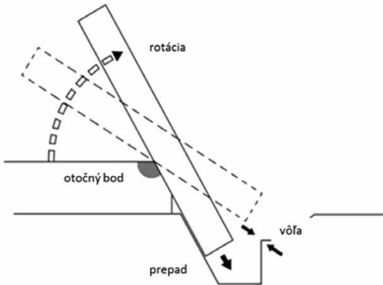
Obr. 3: Spôsob otočenia kameňa na otočnom bode a jeho spustenie do úložnej jamy
